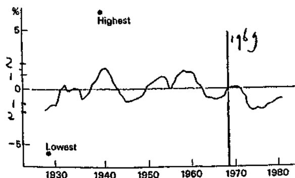
Totale hoeveelheid atmosferische ozon, 1926-1980, gemeten in Arosa, Zwitserland (2).
